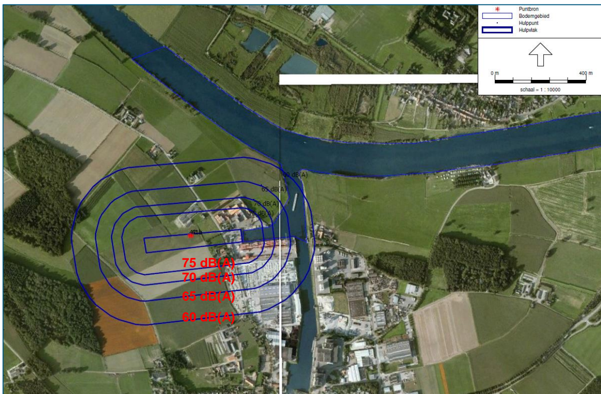
Figuur 3.7: Geluidcontouren a.g.v. het intrillen van damwandplanken
